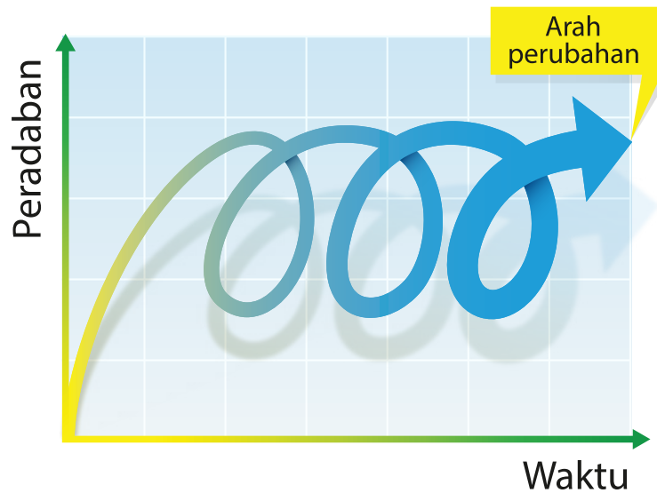
Gambar 1.8 Ilustrasi proses perubahan siklus
