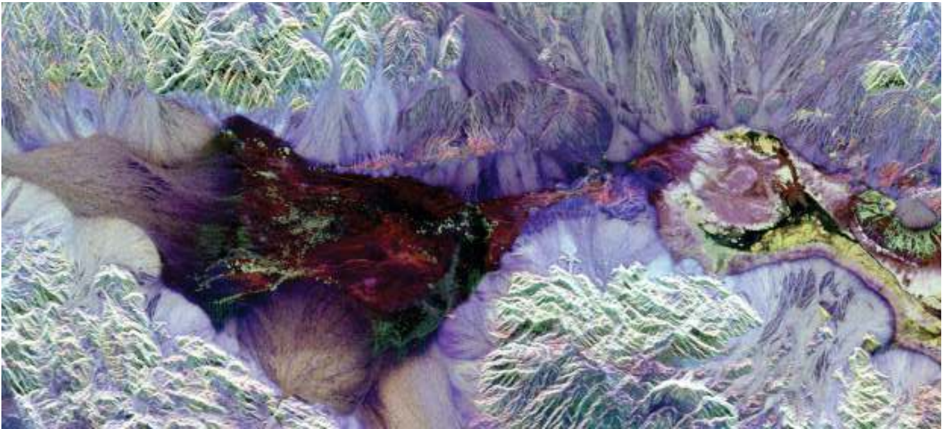
Gambar 2.9 Citra Death Valley, California, dengan polarimetri dilihat dari instrumen radar apertur sintesis pesawat ulang alik
