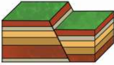
Gambar 3.48 Patahan
