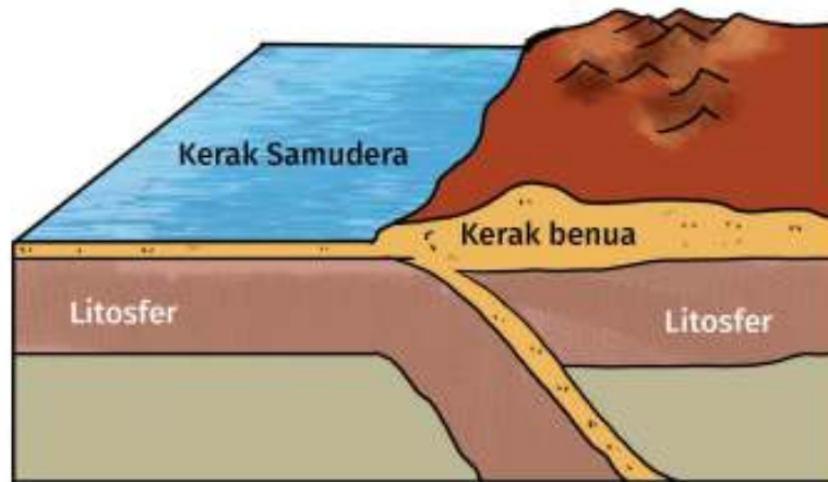
Gambar 3.41 Kerak Bumi
