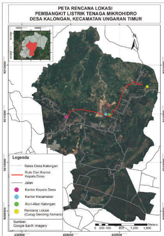
Gambar 2.29 Peta Rencana Lokasi Pembuatan PLTMH
