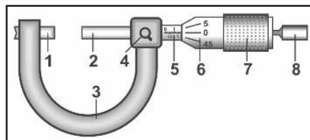
Gambar 1.9. Mikrometer Sekrup
